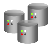
Database
